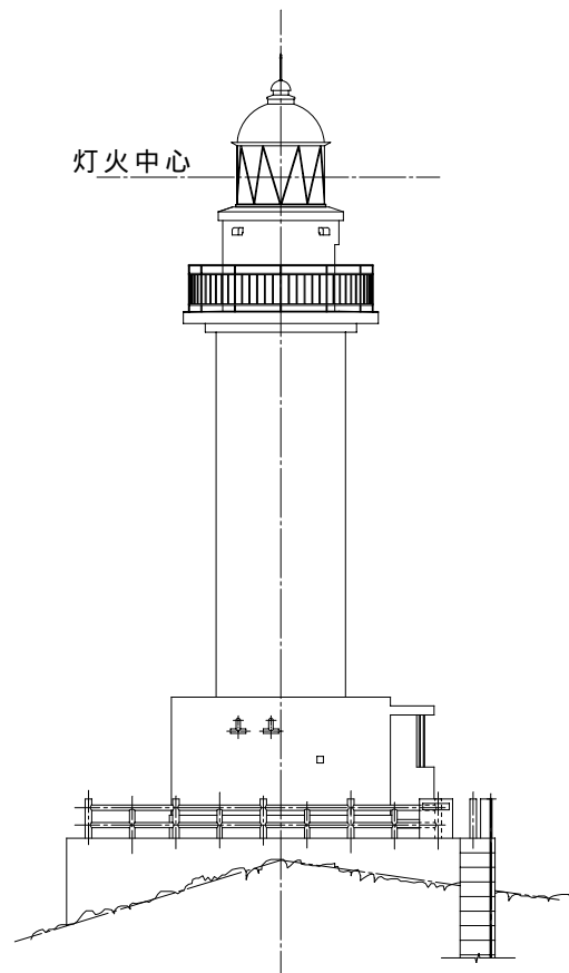
立面図
