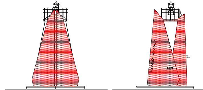
灯台姿図
